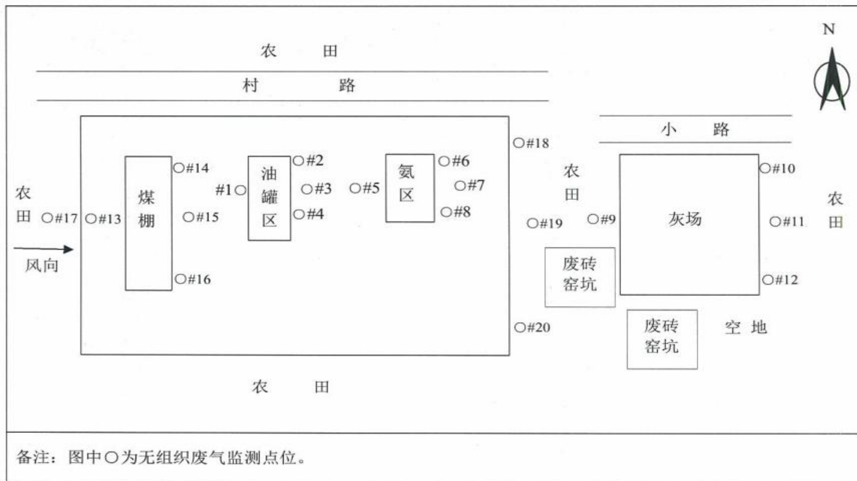
附图 5-1 厂区无组织废气监测布点图
